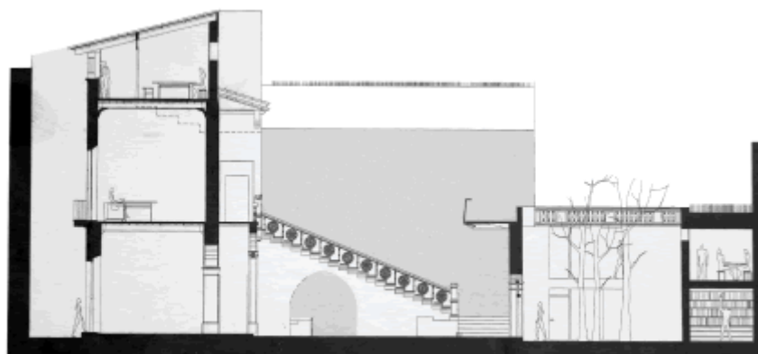
Façana contemporània
